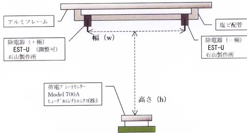
配置図 (+-) 正面視点
