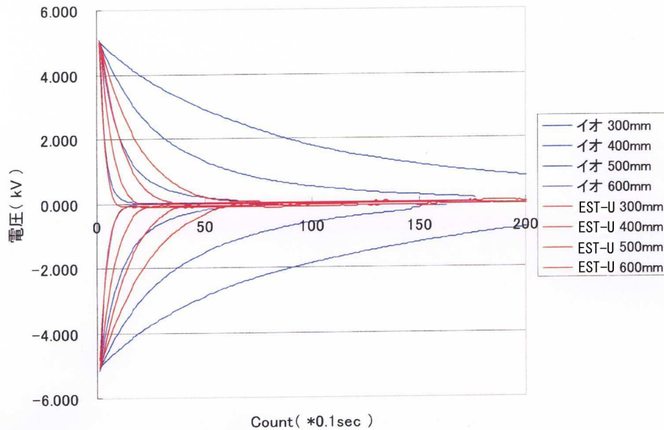
イオナイザーとEST-U 比較 高さ(h)変化による除電時間変化
